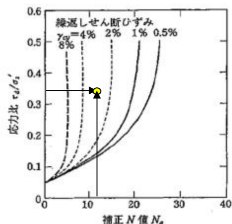
図 4-4 補正 N 値と繰返しせん断ひずみの関係
