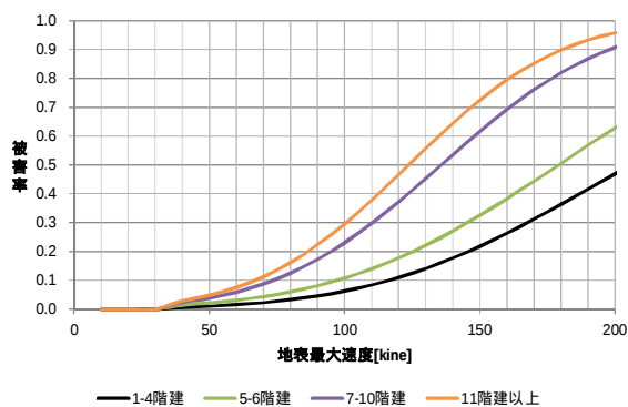
図 1-6 RC 造建物の被害率 (1972-81 年)
