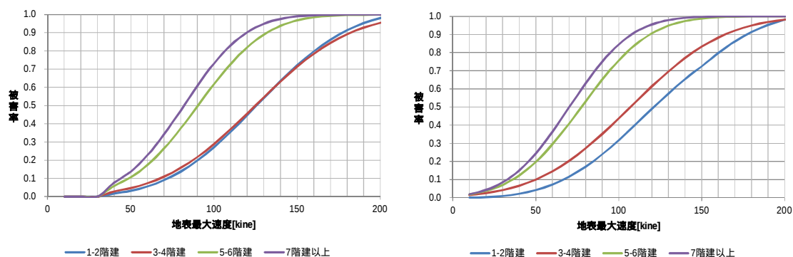
図 1-3 S 造建物の被害率（1981 年以前）
