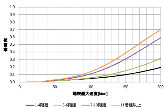
図 1-7 RC 造建物の被害率 (1982 年以後)
