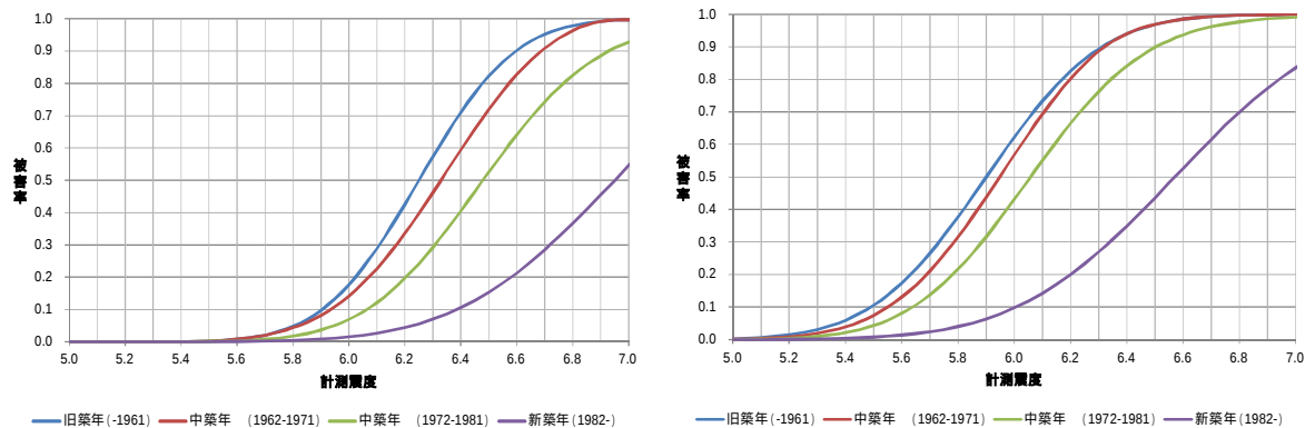
図 1-2 木造建物の被害率
