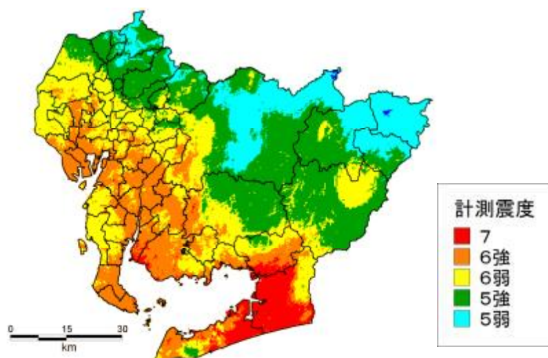
図 3-5 最大想定モデルの地震（東側ケース）による地表震度分布 （統計的グリーン関数法、線形応答計算による）
