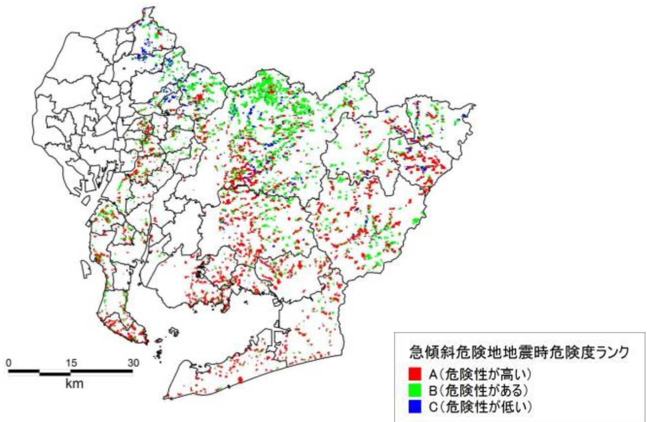
図 5-3(1) 5地震参考モデルの地震における急傾斜地崩壊危険箇所の危険度
