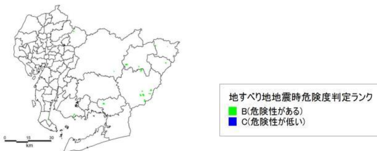
図 5-4(3) 最大想定モデルの地震 (陸側ケース)における地すべり危険箇所の危険度
