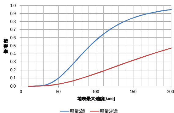
図 1-8 軽量 S 造及び軽量 SP 造建物の被害率
