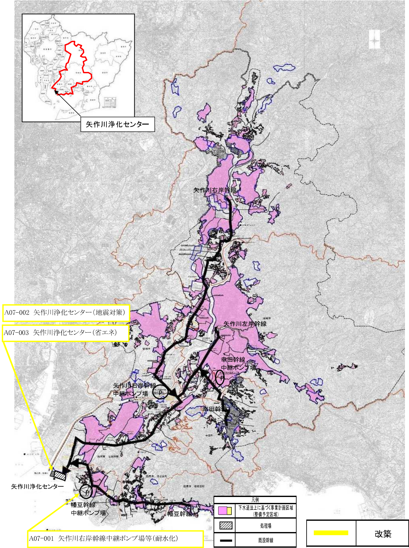
矢作川・境川流域下水道(矢作川処理区)
