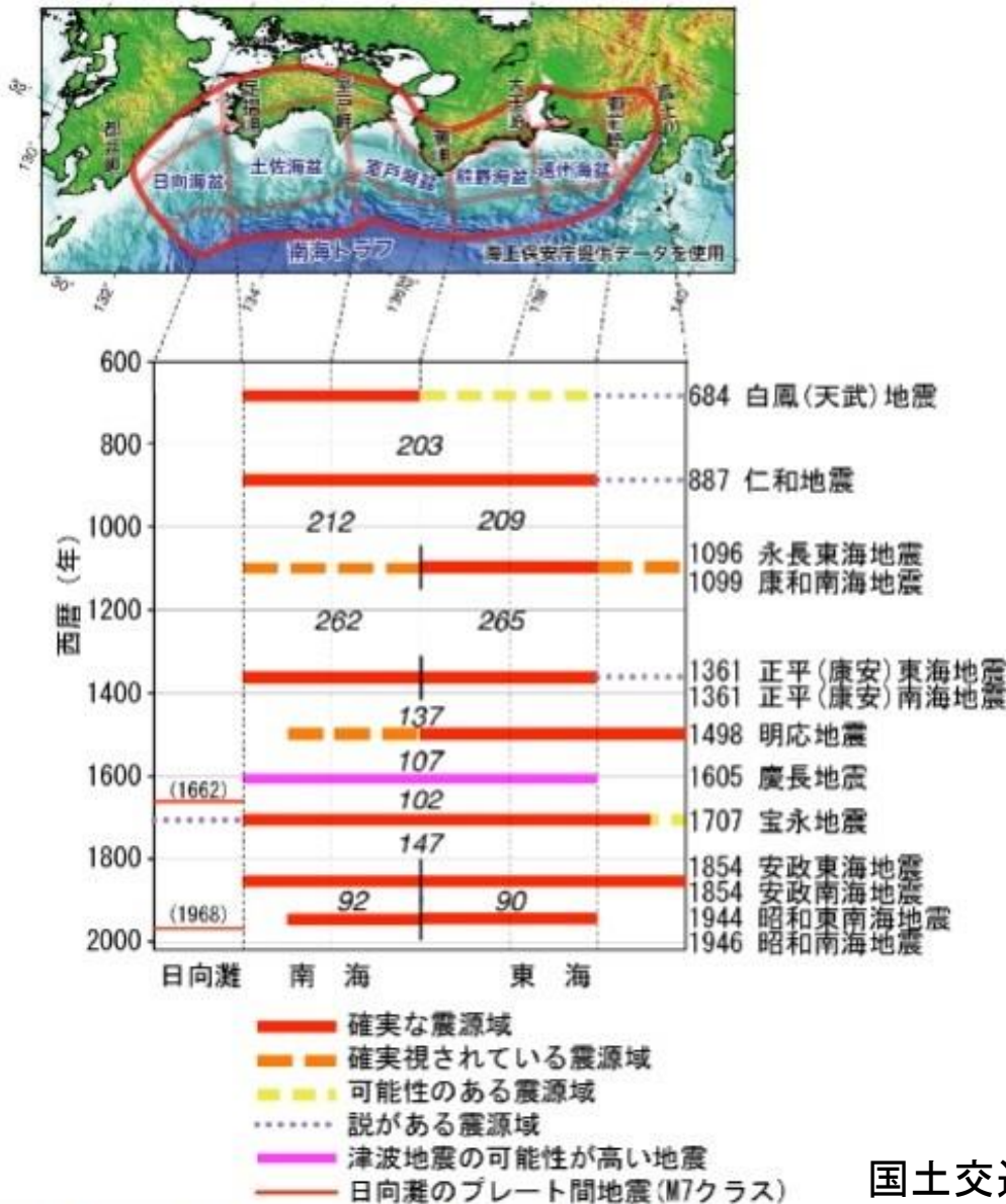
過去に発生した南海トラフ地震の震源域の時空間分布
