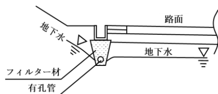
図 3.25 地下排水溝の例
