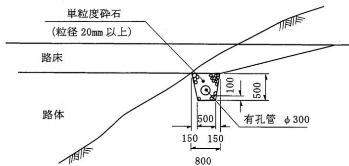
図 3.29 地下排水（切盛境横断排水管）の例
