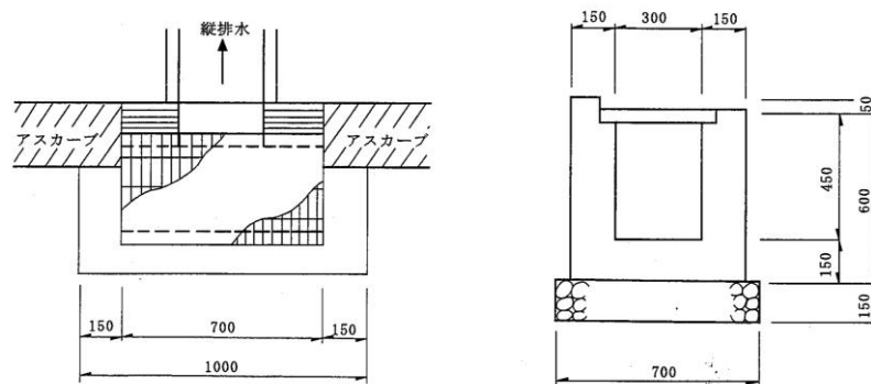
図 3.12 アスカーブに接続する集水柵
