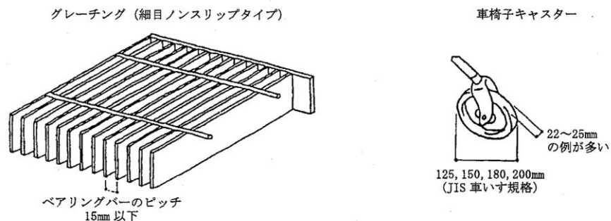
図 3.14 格子蓋 (細目)
