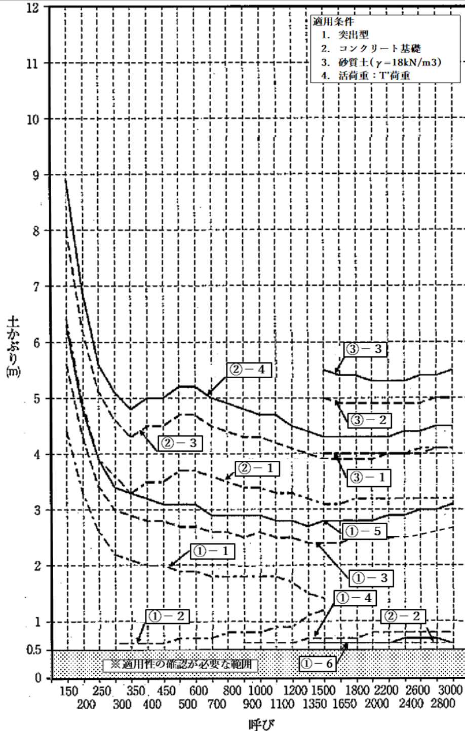
図 4.7 パイプカルバートの基礎形式選定図（遠心力鉄筋コンクリート管，突出型，砂質土）
