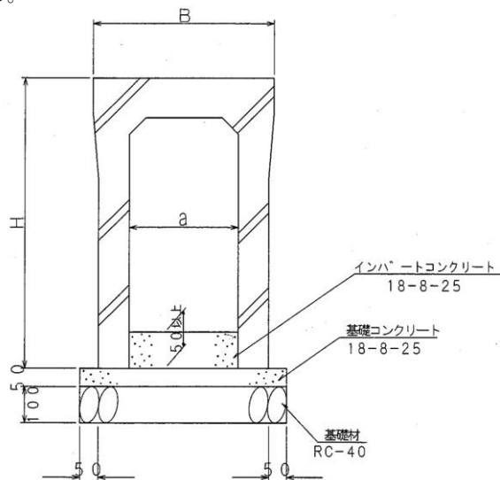
図 3.18 自由勾配側溝
