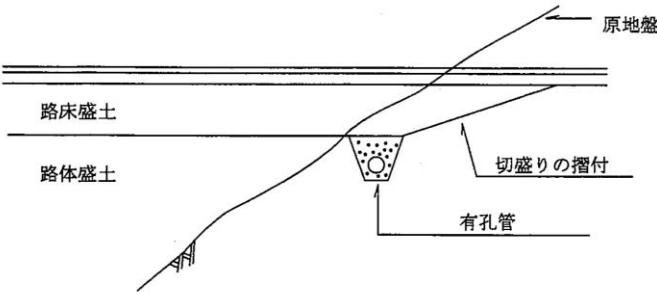
図 3.26 地下排水溝の例
