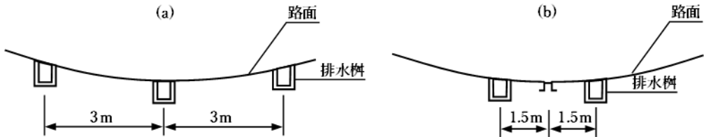
図 3.9 谷部や高架橋の場合の柵配置
