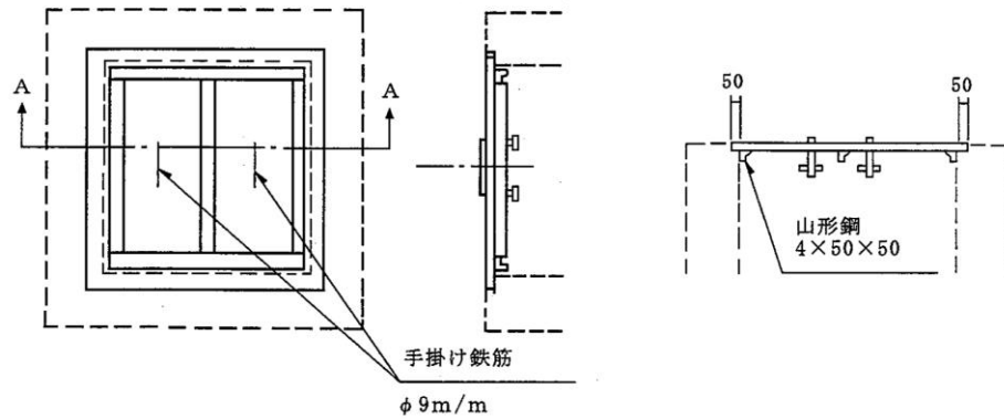
図 3.13 集水桝鋼製蓋
