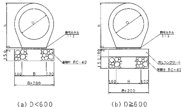
図 4.1 鉄筋コンクリート台付管標準図
