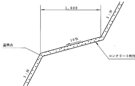
図 3.23 コンクリート吹付のり面の小段
