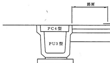
図 3.2 一般部の排水構造
