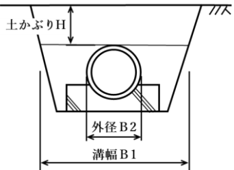
図 4.4 溝型の範囲
