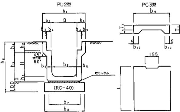
PU2型（道路用プレキャスト鉄筋コンクリートU型側溝：蓋付）寸法および材料表
