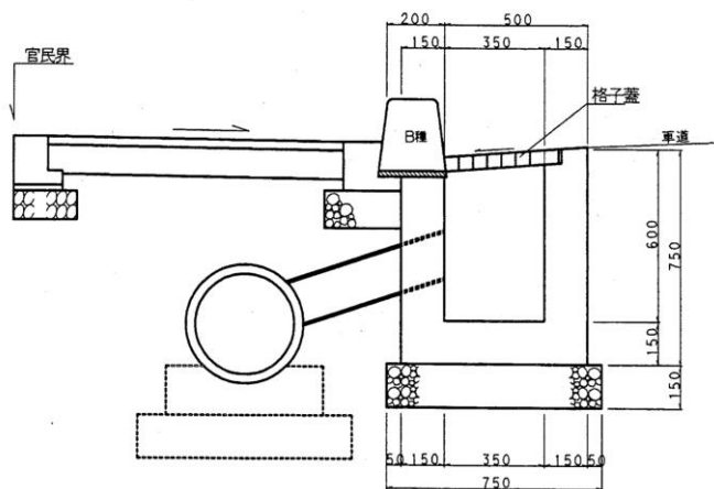
図 3.11 街渠柵の構造
