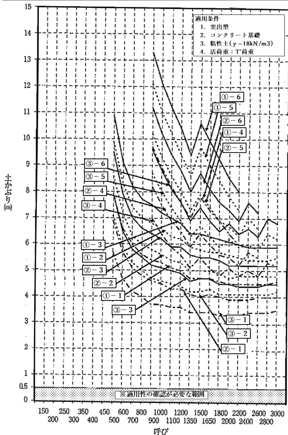
図 4.6 パイプカルバートの基礎形式選定図 (プレストレストコンクリート管, 突出型, 粘性土)
