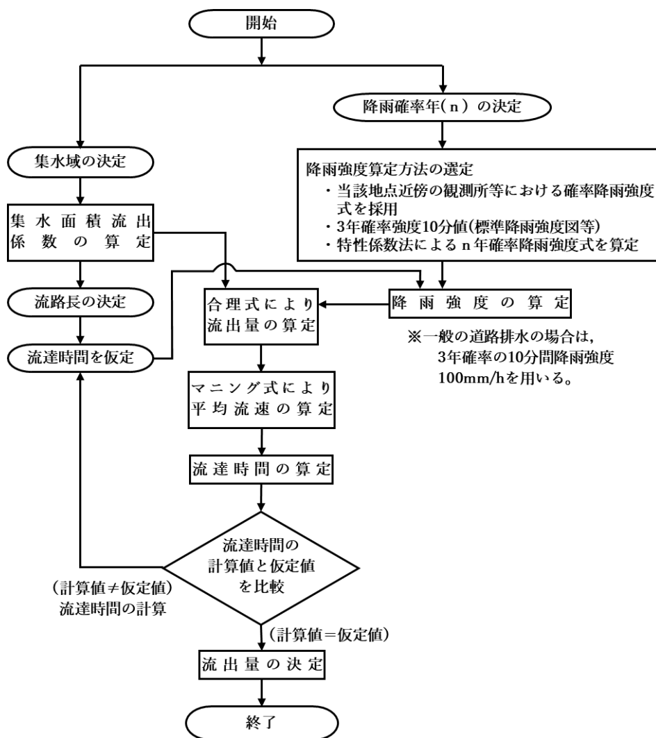
図 2.1 算出手順
