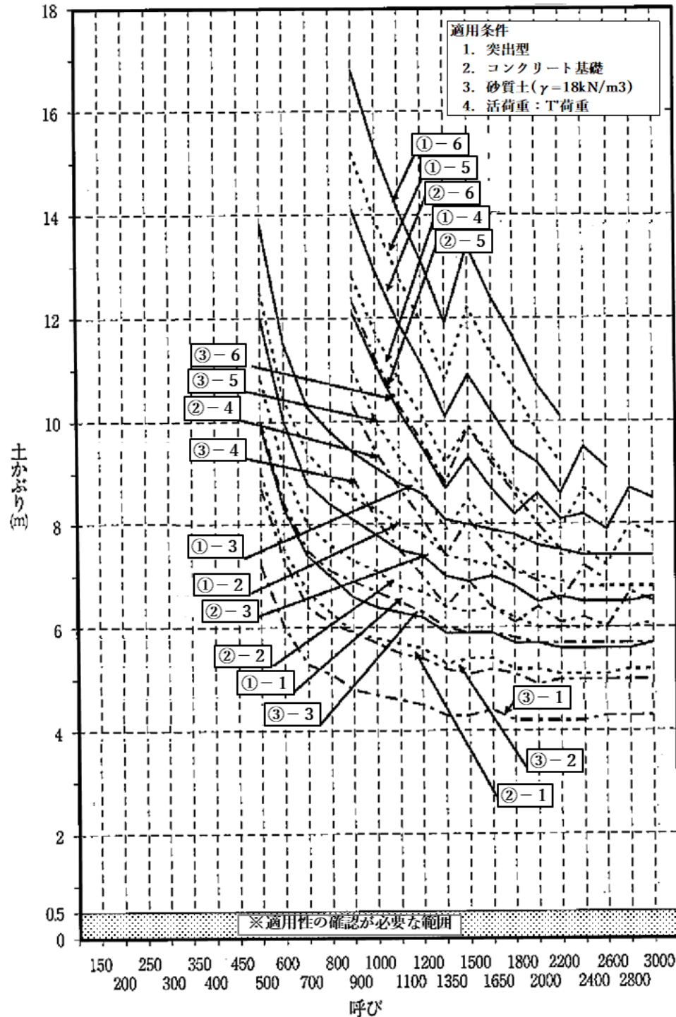
図 4.8 パイプカルバートの基礎形式選定図 (プレストレストコンクリート管, 突出型, 砂質土)
