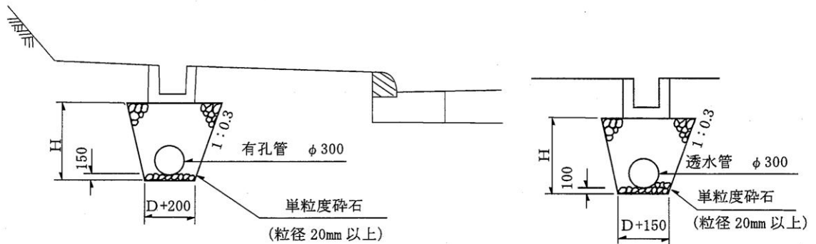
図 3.28 地下排水（縦断方向の排水管）
