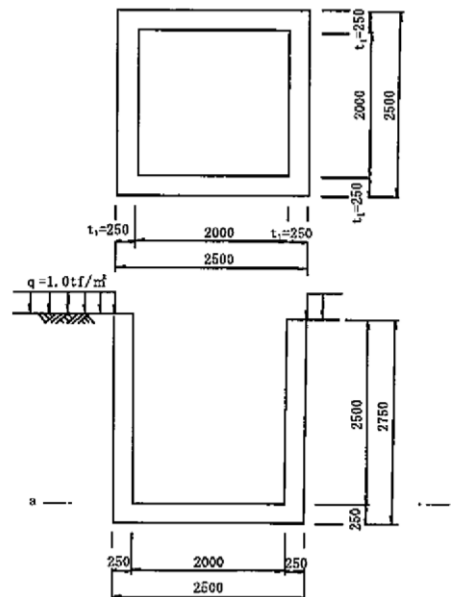
図 5.2 形状
