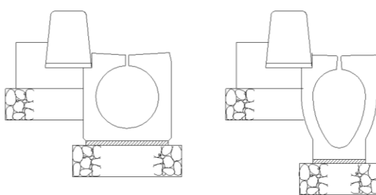
(a) プレキャスト円形水路の例
