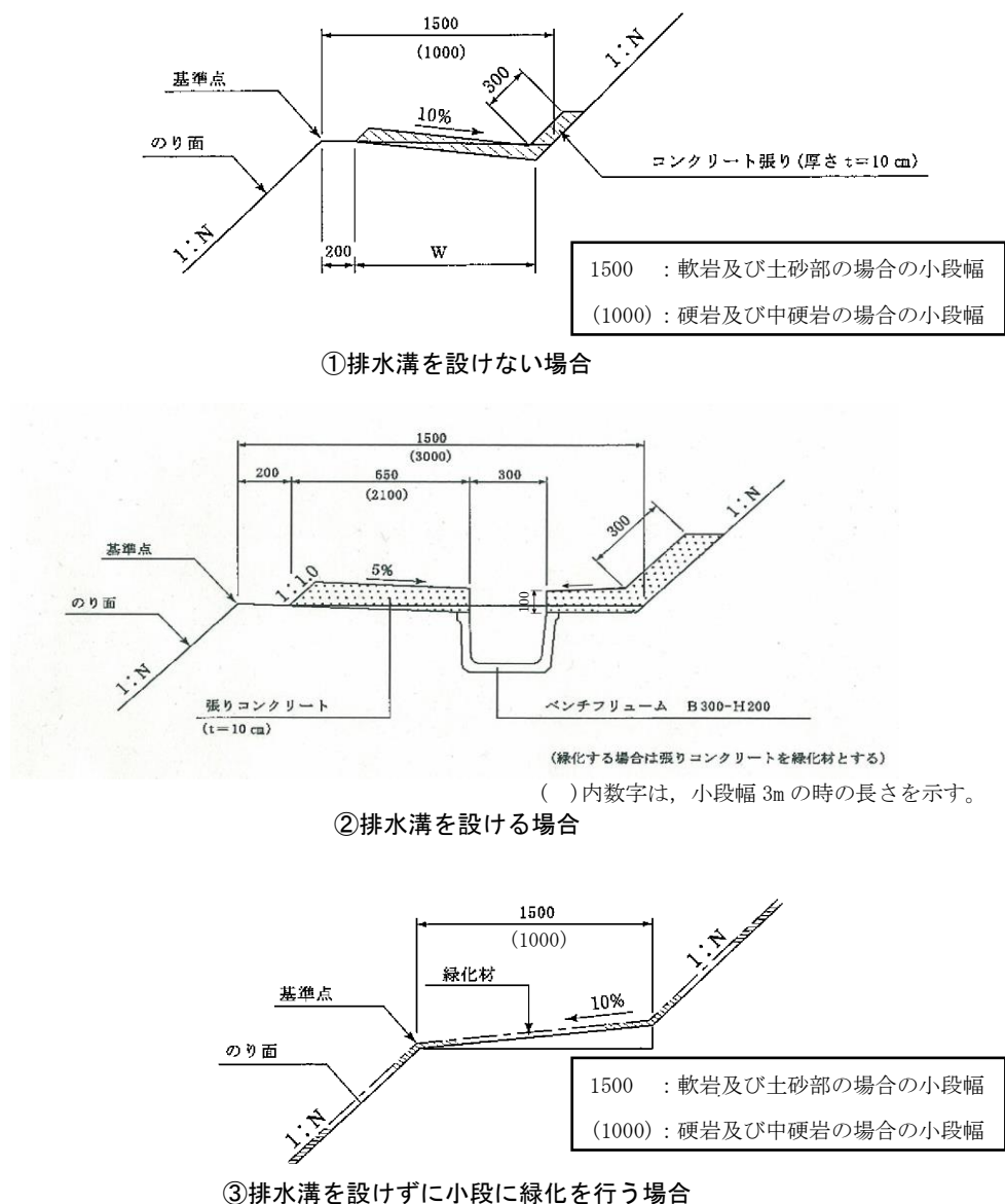
図 3.22 小段排水の構造
