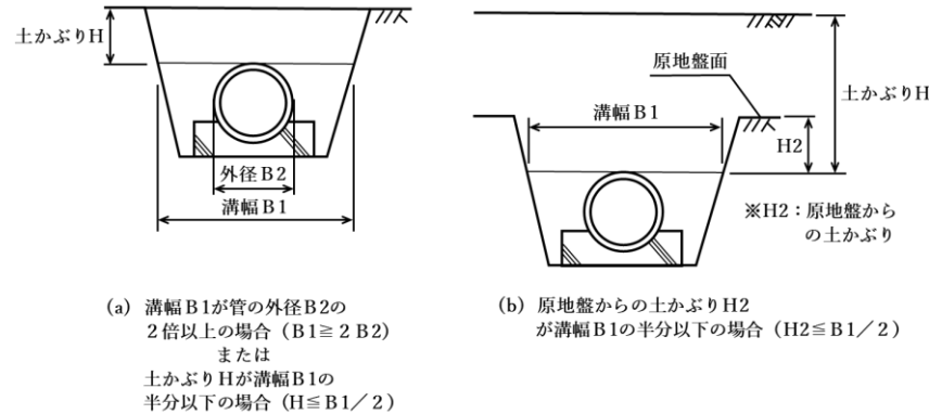
図 4.3 突出型の範囲
