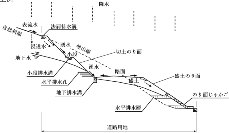
図 3.20 法面排水の施工例
