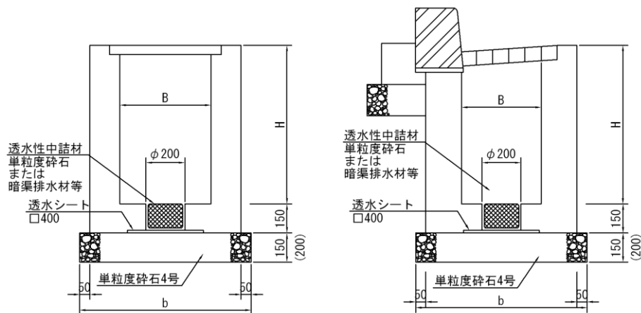
図 3.15 浸透樹の例
