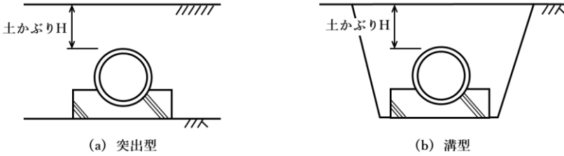
図 4.2 埋設形式
