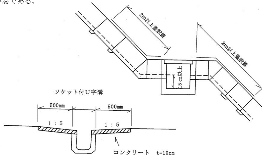
図 3.24 縦排水
