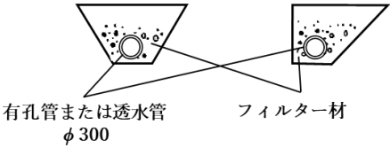
断面例
