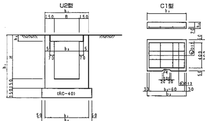
U2型（場所打ちU型側溝：ふた付き）寸法および材料表
