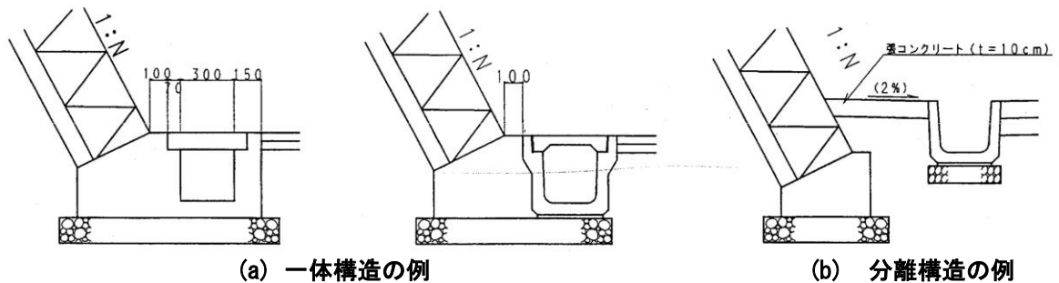
図 3.16 ブロック積擁壁基礎兼用の側溝
