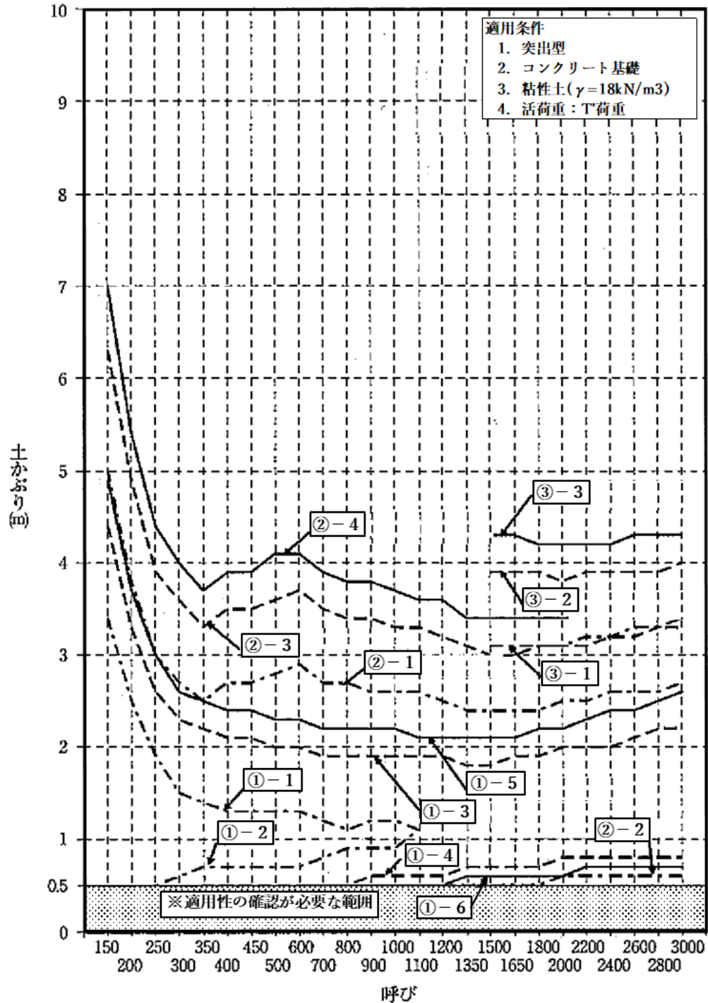
図 4.5 パイプカルバートの基礎形式選定図（遠心力鉄筋コンクリート管，突出型，粘性土）
