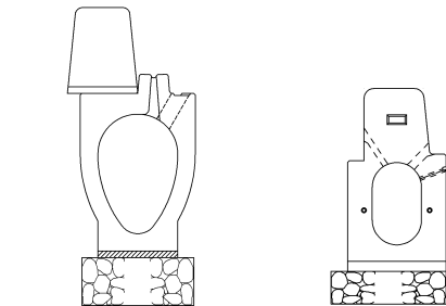
(a') 自転車の走行性に配慮した排水施設の例
