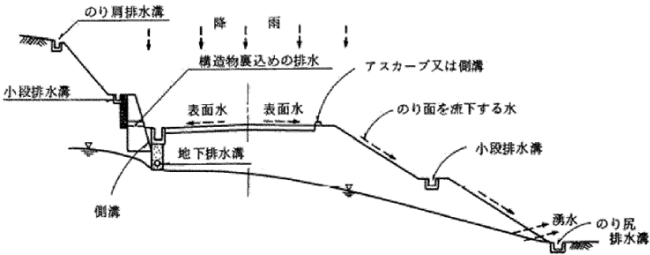
図 1.1 排水の種類
