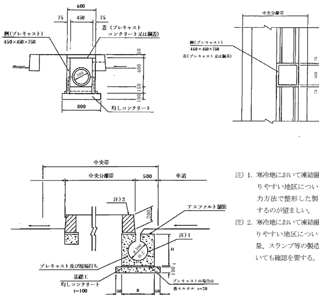
図 3.8 中央分離帯の排水
