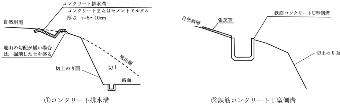
図 3.21 法肩排水の種類
