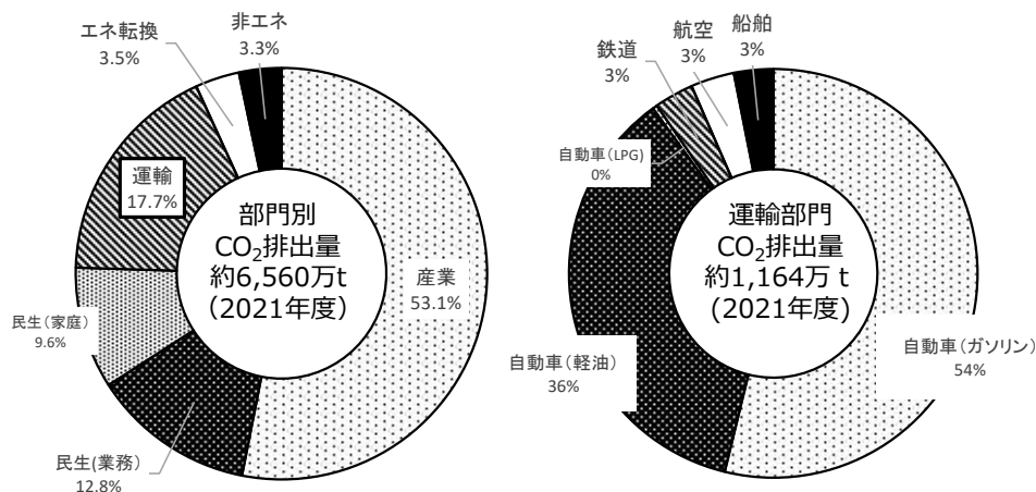
図9 愛知県内の二酸化炭素排出量に占める運輸部門の割合（2021年度）
