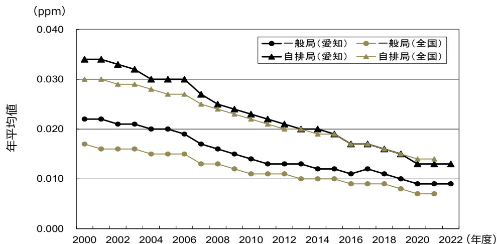
図3 二酸化窒素の濃度（年平均値）の推移
