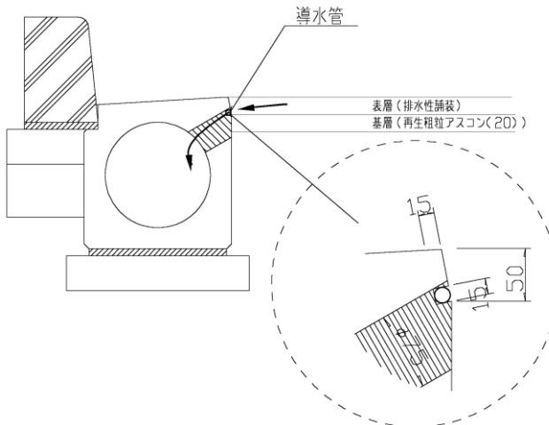
図 3.18 箱型パイプの事例
