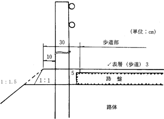
図 5.11 転落防止柵
