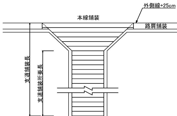
図 9.2 歩道のない場合
