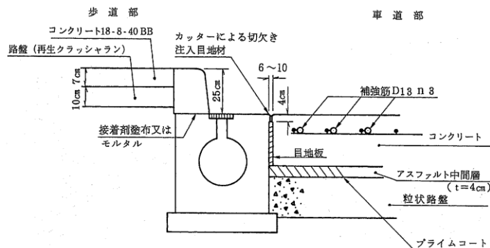
図 4.2 端部の構造
