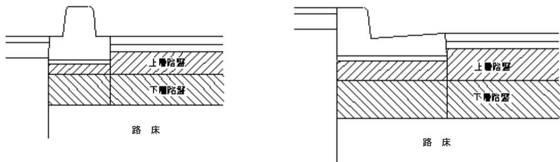
図 5.9 境界ブロック下部の施工
