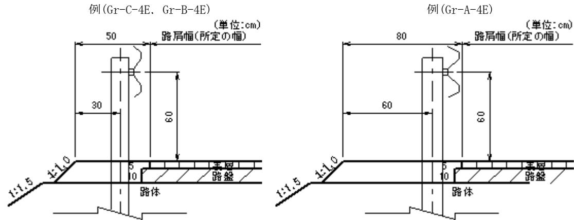
図 5.10 ガードレール
