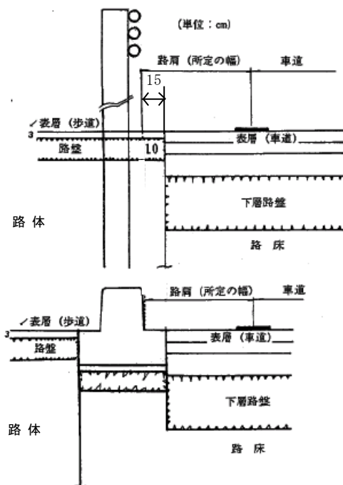
図 5.8 ガードレール分離
