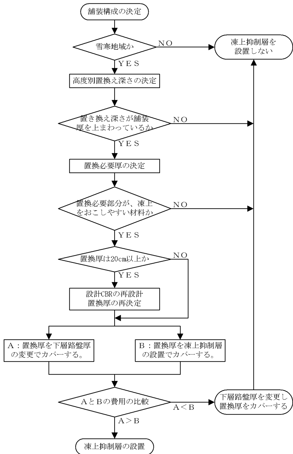
図 3.10 凍上抑制層設計手順
