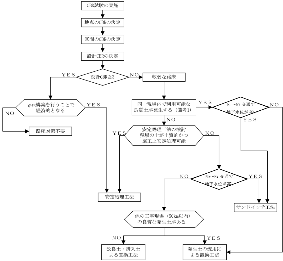
図 3.7 工法選定手順
