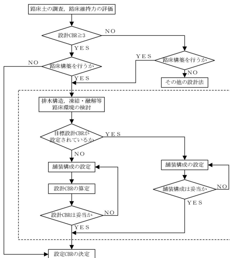
図 3.5 路床の設計手順
