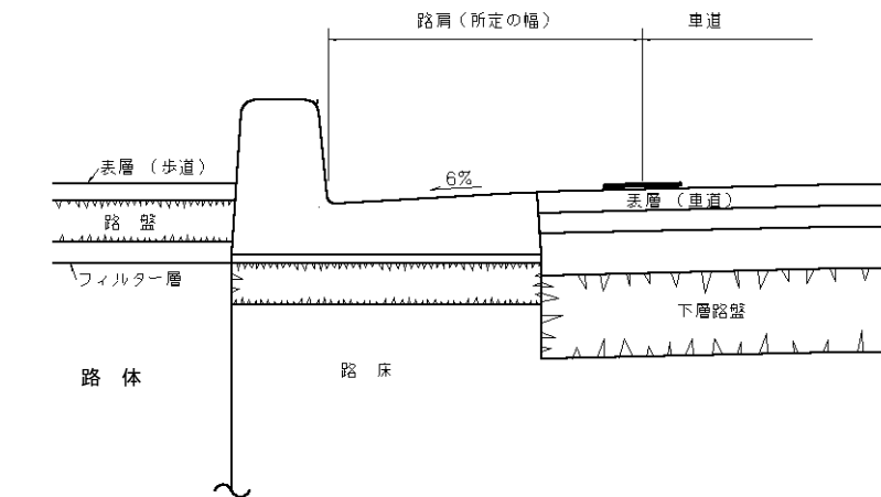
図 5.6 歩道を設置する場合
