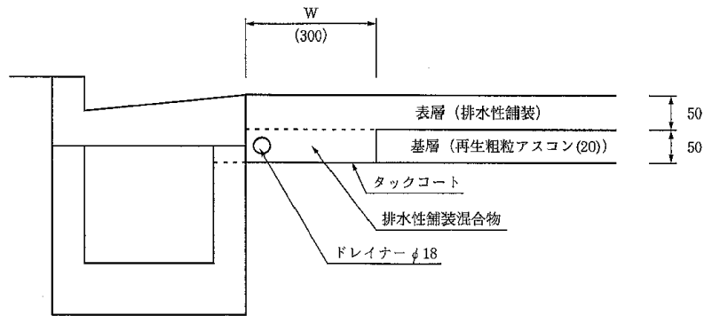
図 3.16 舗装端部の排水構造
