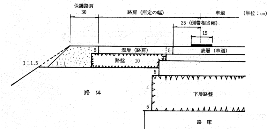
図 5.5 歩道を設置しない場合
