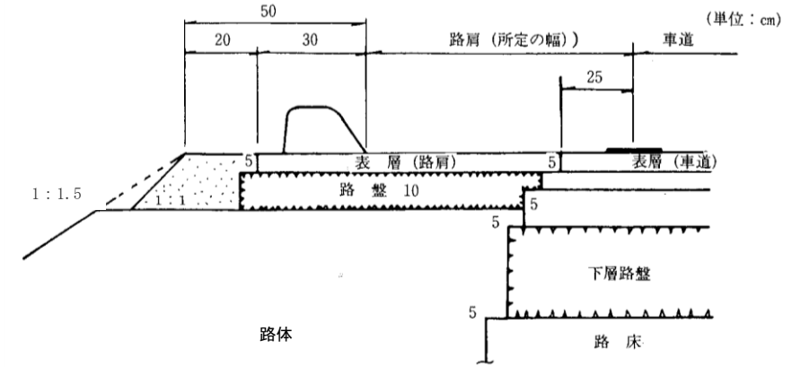
図 5.12 アスカーブ
