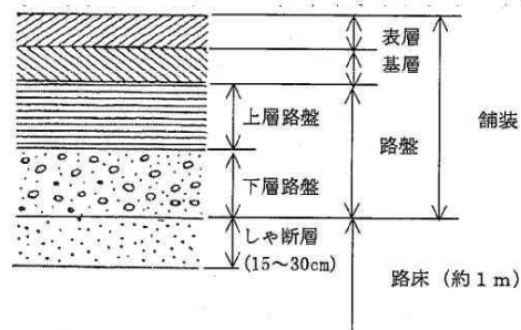
図 3.9 舗装の構成
