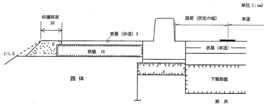
図 5.7 ブロック分離
