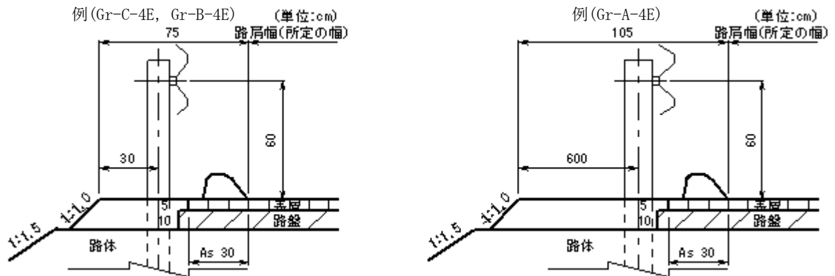
図 5.13 アスカーブとガードレールを併設する場合
