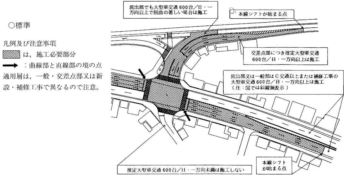
図 3.11 交差点部(標準)
