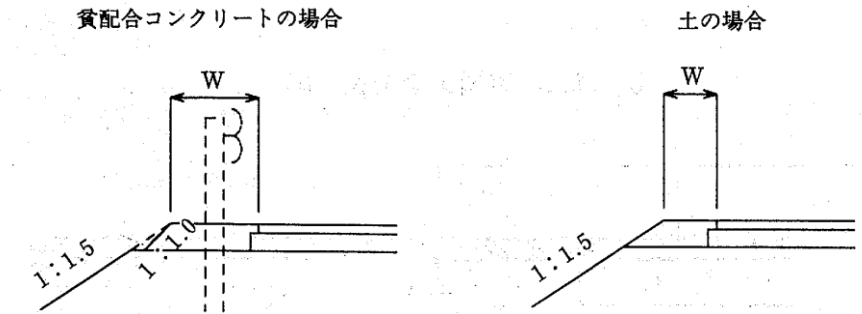
図 5.4 保護路肩処理
