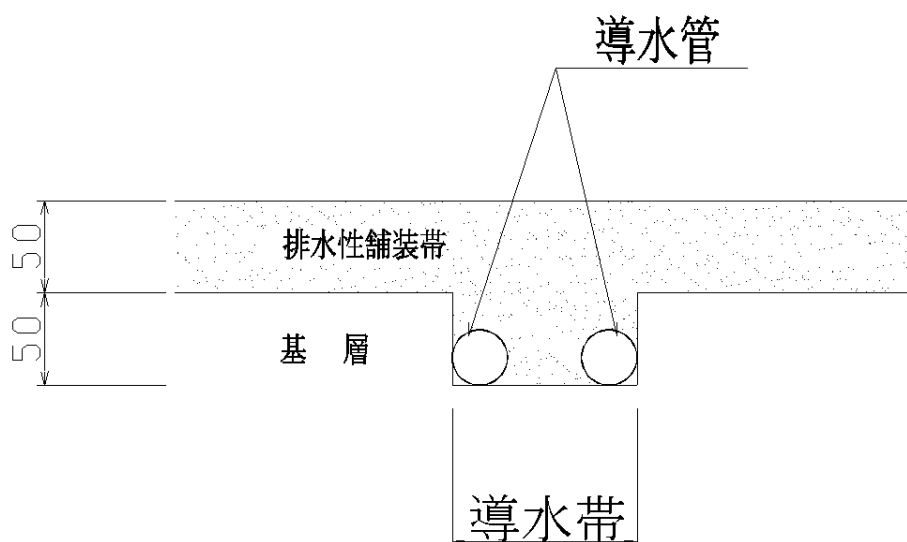
図 3.14 合成勾配方向の導水帯断面図(例)
