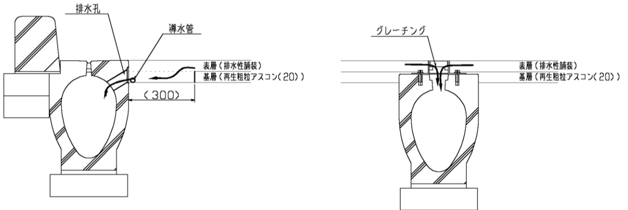
図 3.17 卵形側溝の事例
