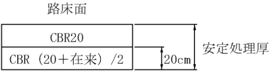
図 3.8 CBR の計算法
