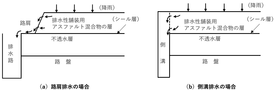
図 3.15 標準的な舗装構成例(矢印は雨水の流れ)
