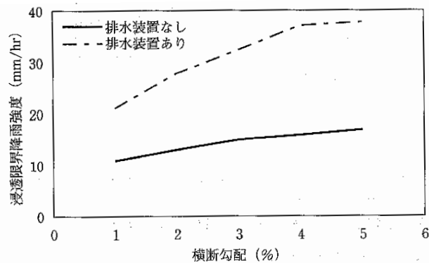
図 3.19 横断勾配に対する表面流出しない降雨強度の関係
