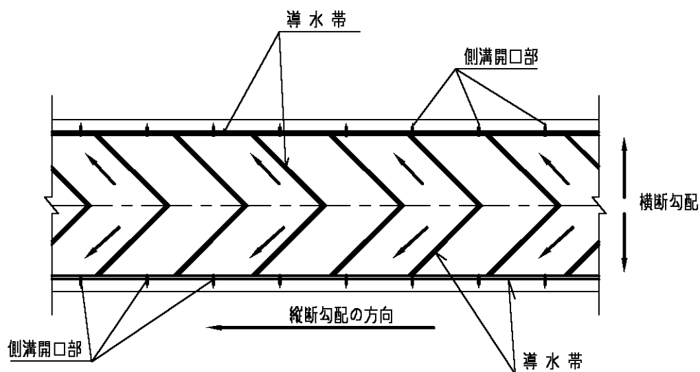
図 3.13 平面図(例)
