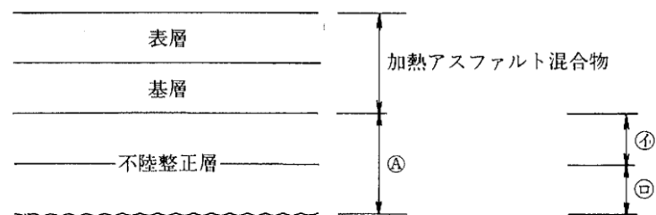
図 3.20 岩盤上の舗装構成
