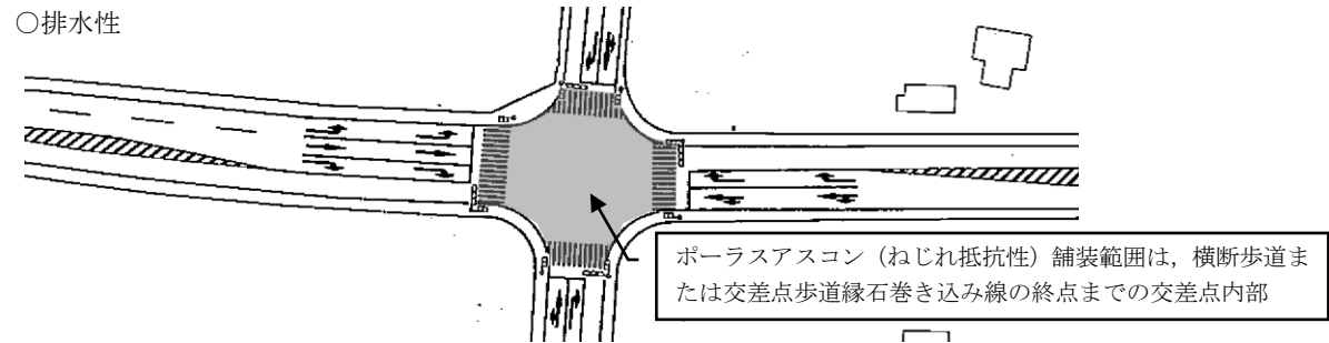
図 3.12 交差点部(ポーラスアスコン(ねじれ抵抗性))
