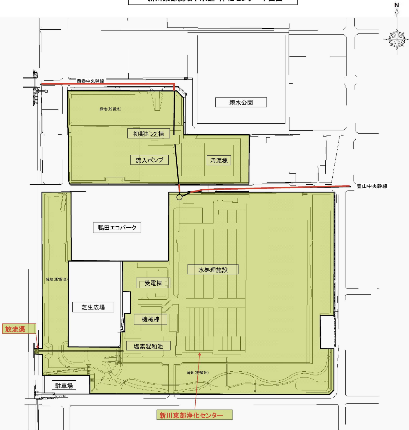
新川東部流域下水道 浄化センター平面図
