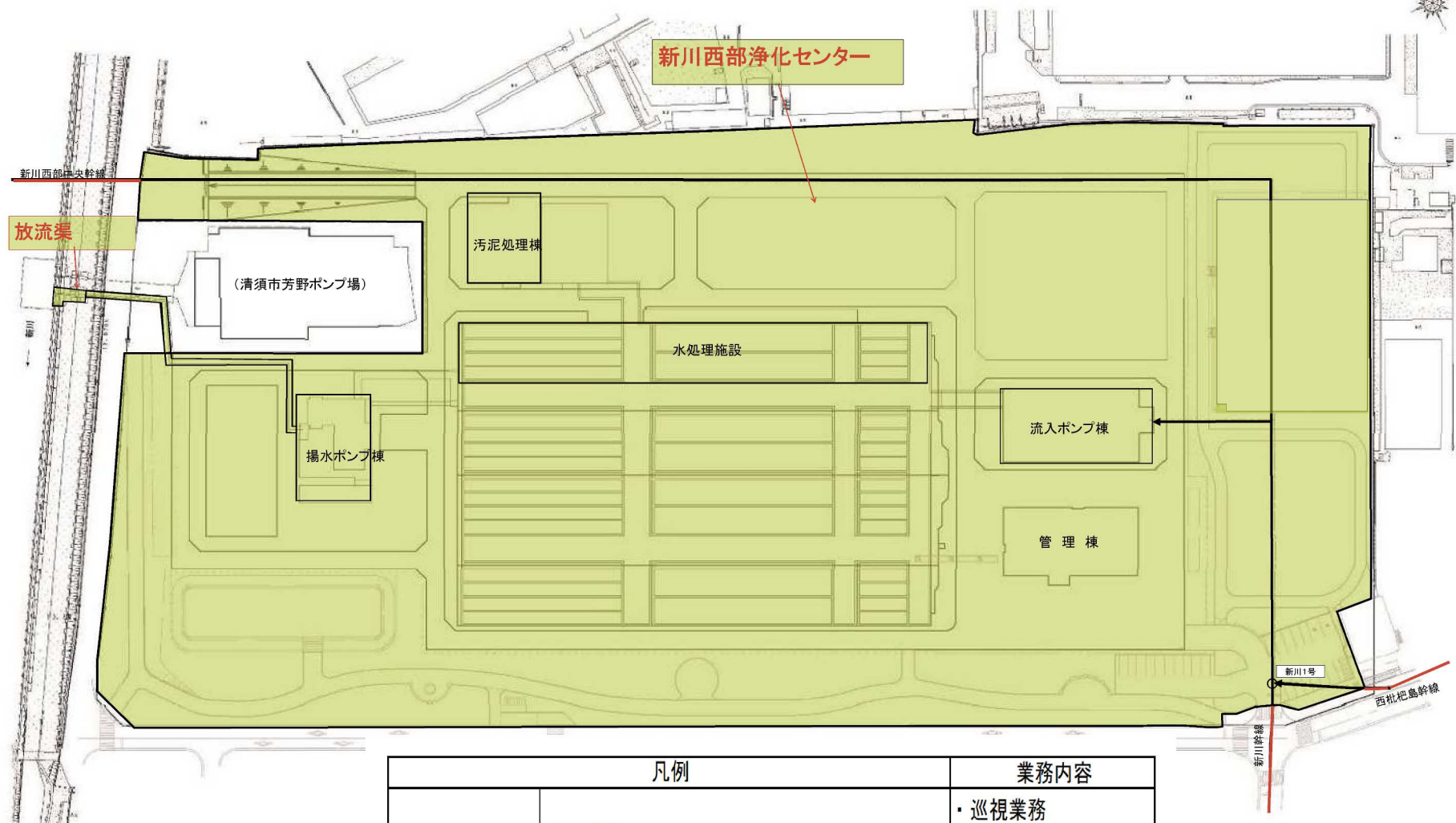
新川西部流域下水道 浄化センター平面図
