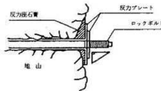
図 4-2 反力座の設置
