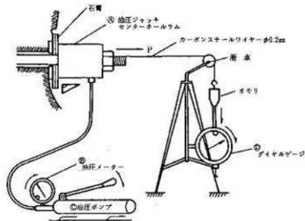
図 4-3 引抜試験装置
