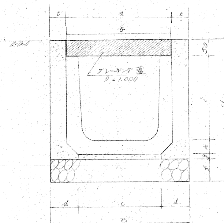
寸法表
