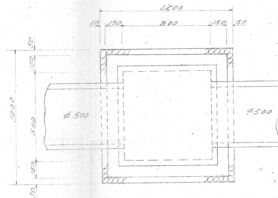
柵 B 型 (0.80x0.80x1.0)
