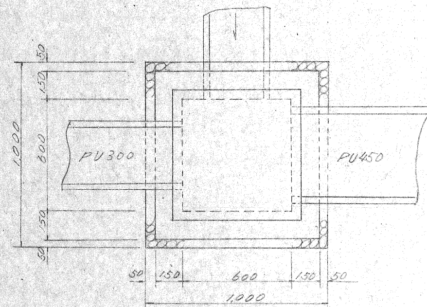
柵 A 型 (0.60x0.60x0.80)
