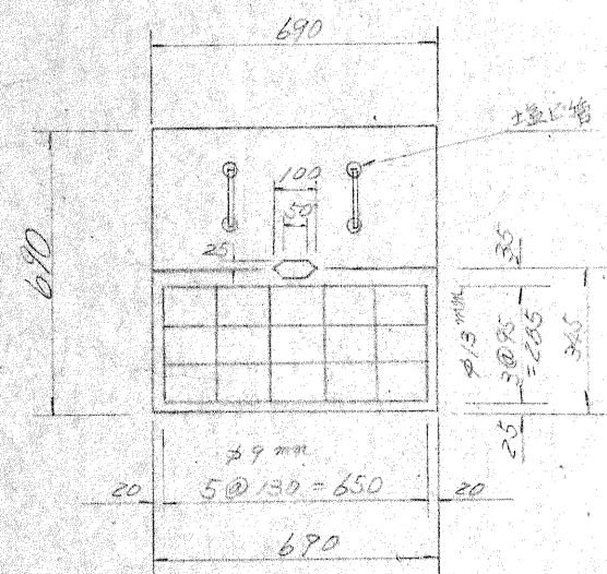
柵 A 型 断面図
