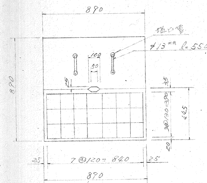
柵 B 型 断面図
