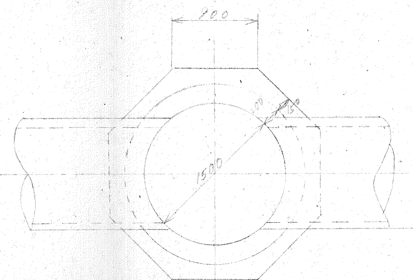
平面圖 S: 1/40
