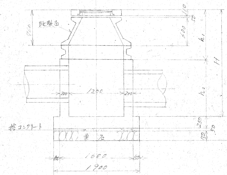
横断面図 S: 1/40
