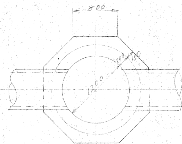
平面圖 S. 1/40
