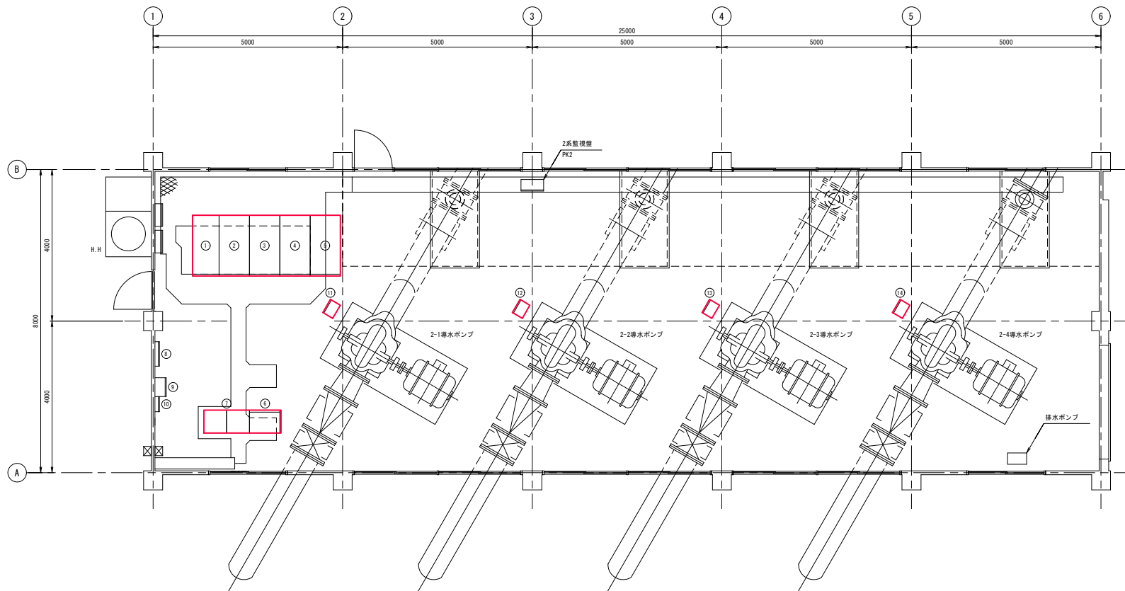
2系導水ポンプ室 平面図 S=1/50
