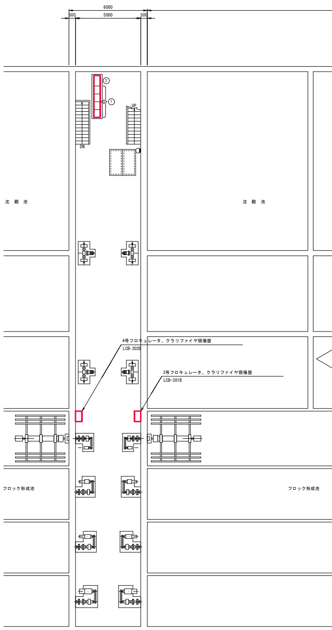
2系上水沈殿池地下1階 平面図 S=1/100
