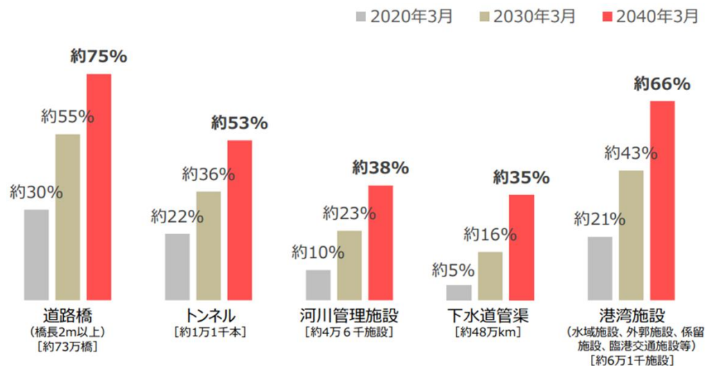
【図表11】建設後50年以上経過する社会資本の割合(全国)
