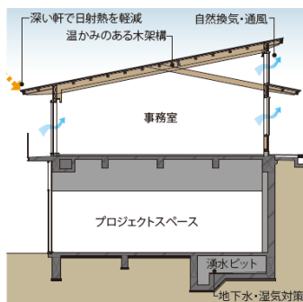
▲交流棟構造
