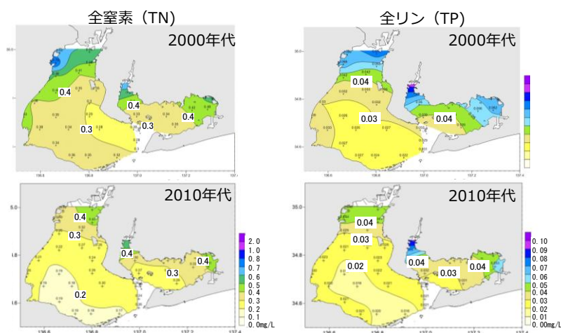
図3-1 伊勢・三河湾における全窒素(TN)及び全リン(TP)の水平分布 1)
