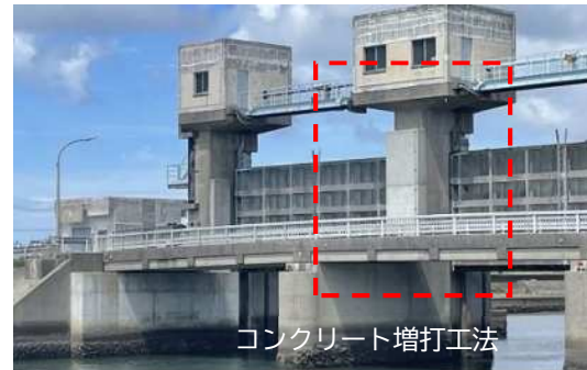
コンクリート増打工法 海岸水門の耐震化 (福江港海岸)
