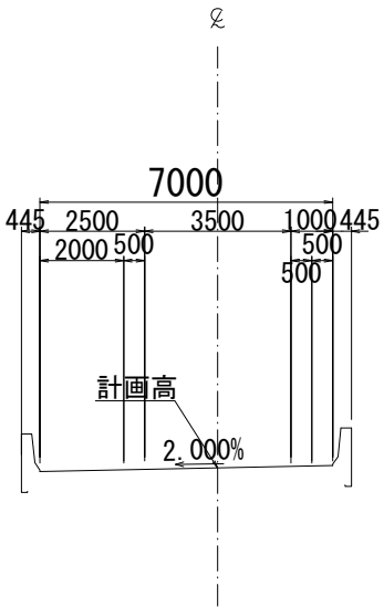
嵩上式(橋梁部)
