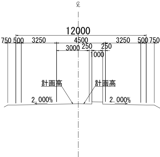
地表式(交差点部)
