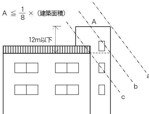
【図1】階段室
