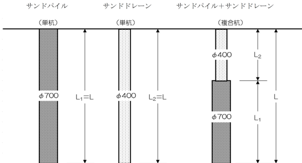
図 6-2 施工図
