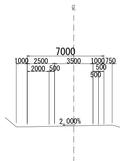
嵩上式(土工部)
