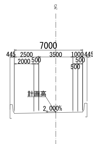
嵩上式(橋梁部)
