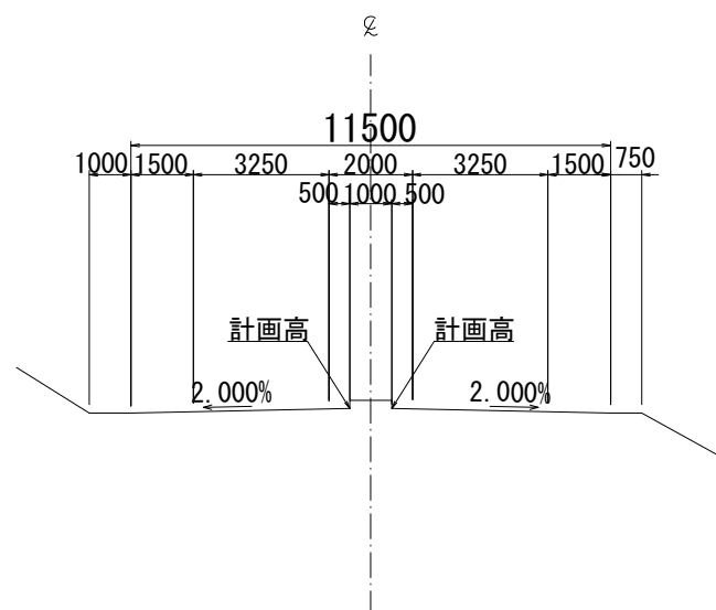
地表式・嵩上式(土工部)
