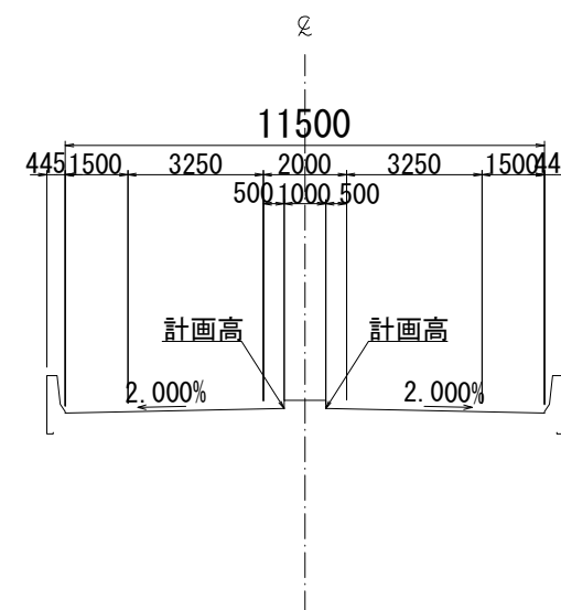
嵩上式(橋梁部)
