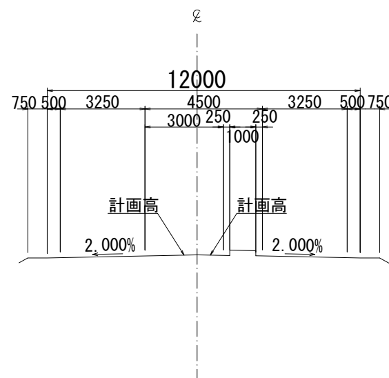
地表式(交差点部)
