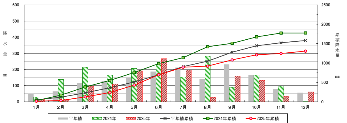
資料図 6－1 名古屋地方気象台における月別降水量と累積降水量
