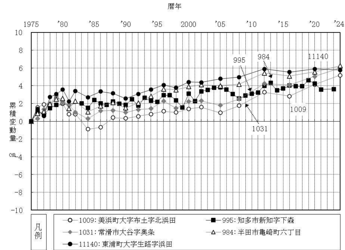
資料図 7－1 主要な水準点の累積変動状況 (2024 年：知多地域)
