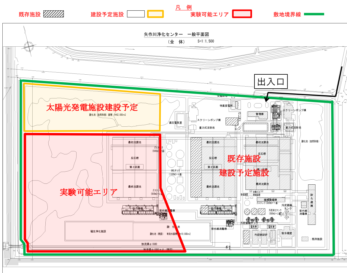
図1 矢作川浄化センター 平面図
