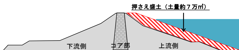
堤体補強断面図
