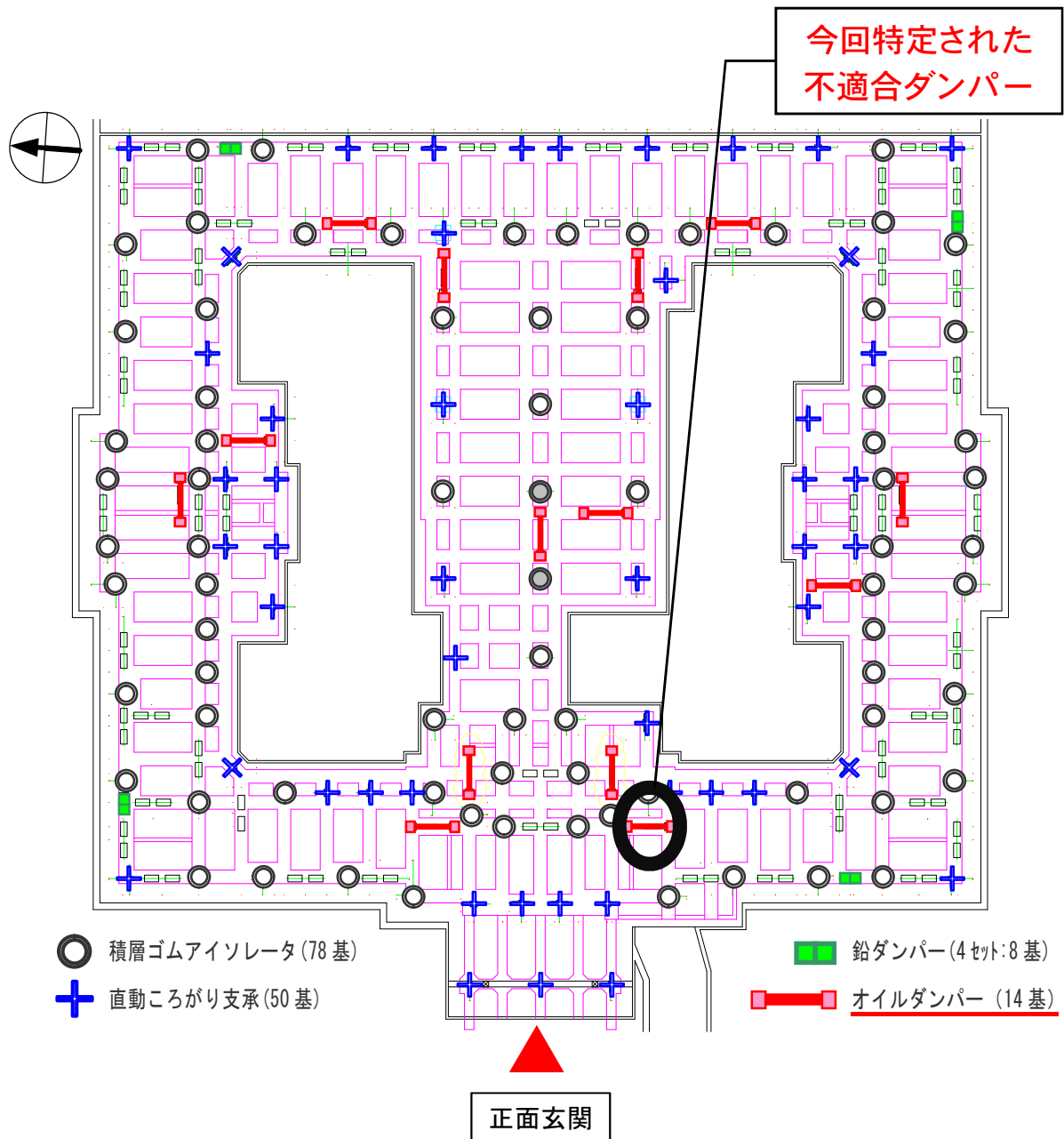
【県庁本庁舎に設置されている免震装置配置図】
