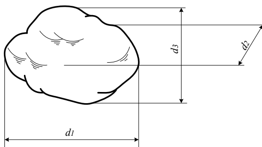
図1-2-8 巨礫の粒径
