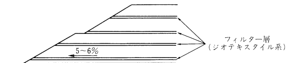
(ジオテキスタイル系のものをういた例)
