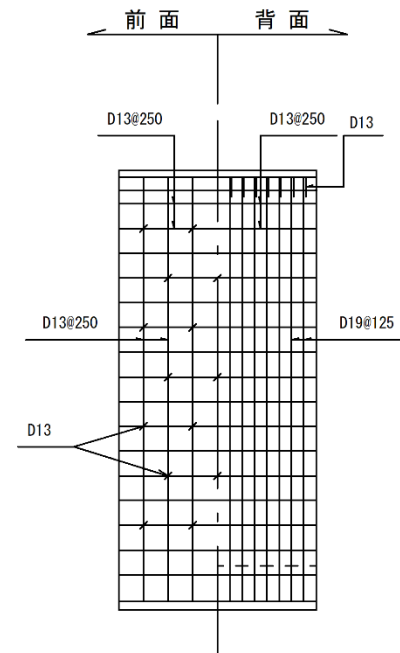
豎壁配筋圖
