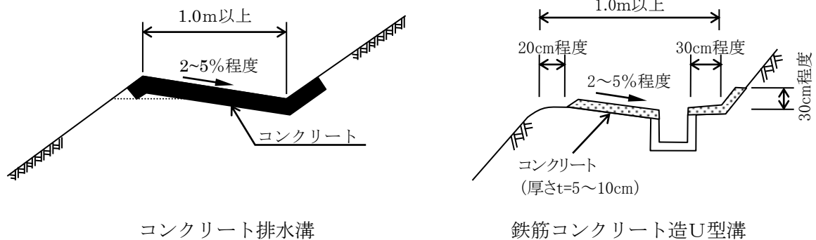
図4-6 小段排水溝の設置例
