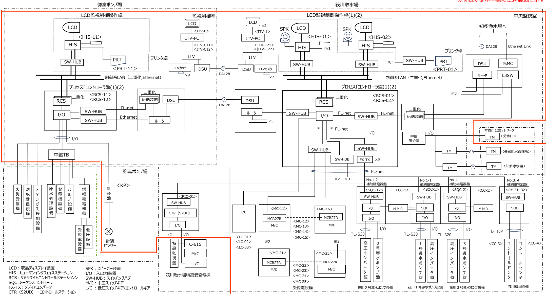
弥富ポンプ場・筏川取水場 監視制御設備システム構成図
