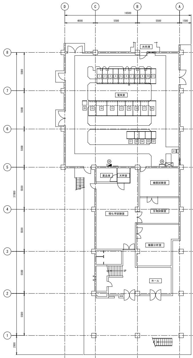
新電気室 平面図 S=1/100
