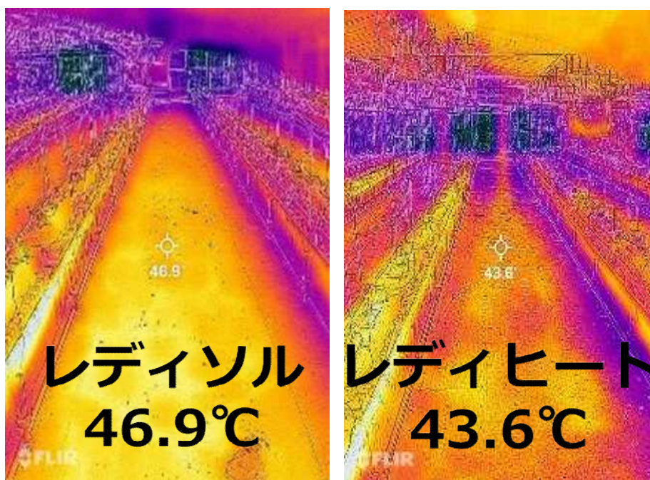
サーモカメラによる遮光剤・遮熱剤の比較
