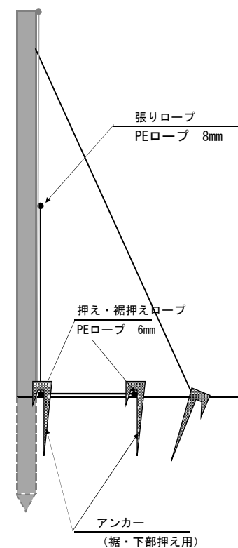
【側面図】
