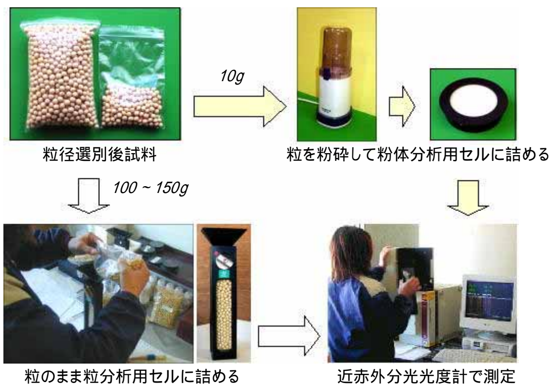
図 -2-2-2 近赤外分光光度計によるダイズの成分分析手法
